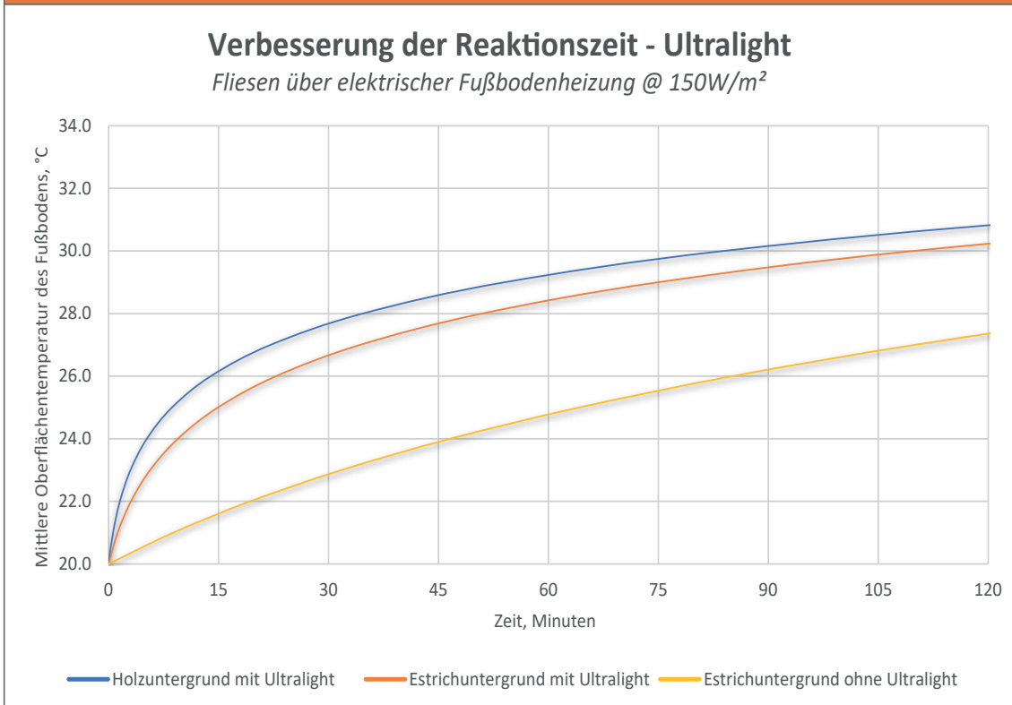
Abbildung 2 - Verbesserung der Reaktionszeit durch den Einsatz von Ultralight Bei Tests mit einer elektrischen Fußbodenheizung von 150 W/m 2 über einem 65 mm isolierten Estrich benötigt der Boden 110 Minuten, um 27°C zu erreichen. Durch die Verlegung von Ultralight unter der elektrischen Fußbodenheizung wird die gleiche Temperatur in nur 34 Minuten erreicht.
