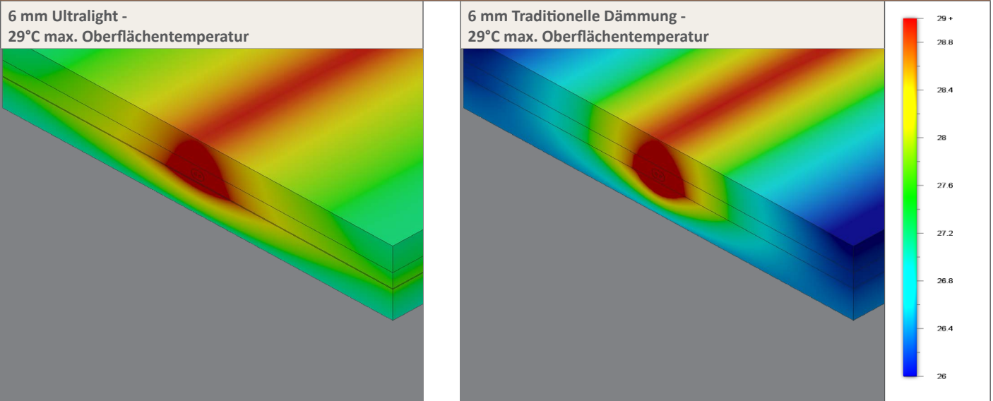
Abbildung 1 - Verbesserte Wärmeausbreitung der Ultralight im Vergleich zu herkömmlicher Dämmung Bei einer maximalen Oberflächentemperatur von 29 °C würde eine herkömmliche Dämmung zu einer minimalen Oberflächentemperatur von knapp unter 26 °C führen. Im Vergleich dazu erhöht der Ultralight die Oberflächentemperatur auf 27,5 °C, was zu mehr Komfort und eine um 10,5 % höhere Heizleistung führt.
